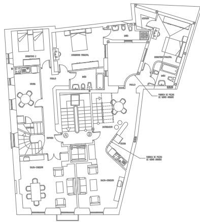
Planta Segunda
