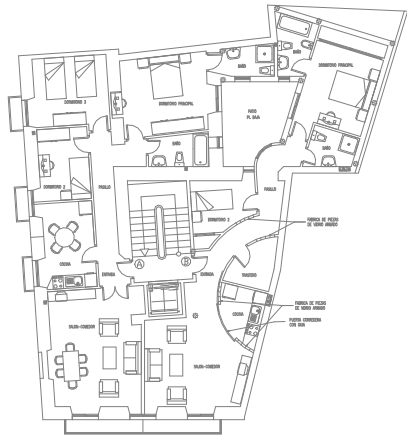
Planta Primera
