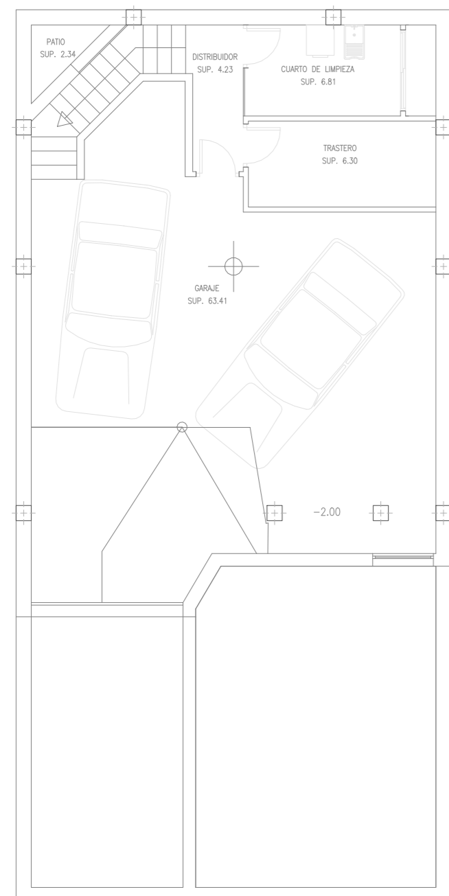
SEMISÓTANO
