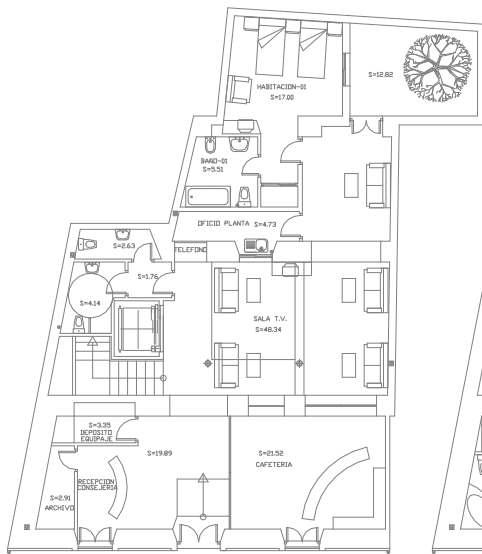
PLANTA PRIMERA
