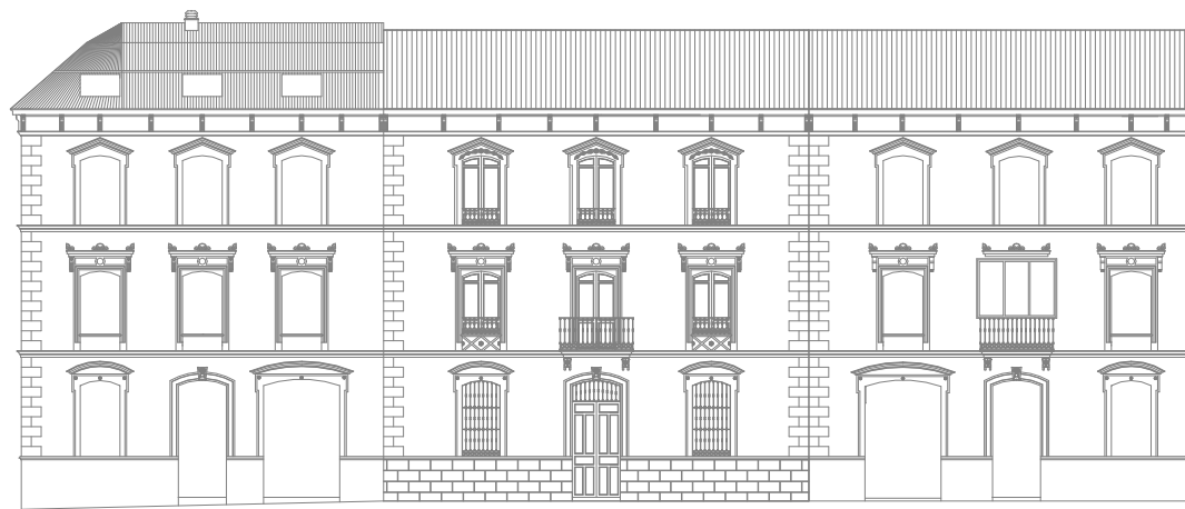
ALZADO
