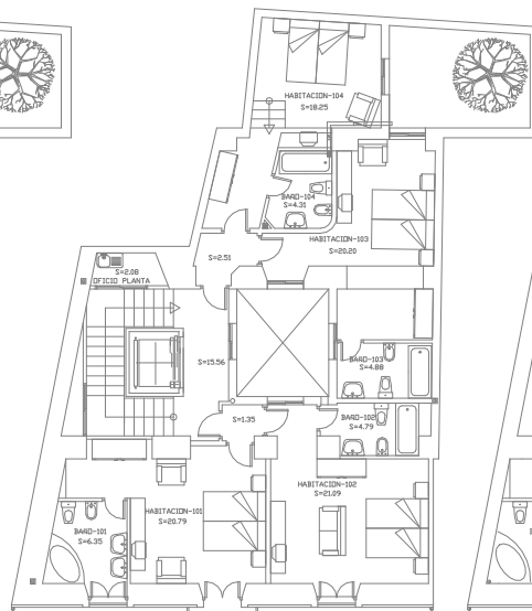
PLANTA SEGUNDA
