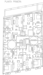
PLANTA PRIMERA
