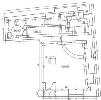
PLANTA BAJA
