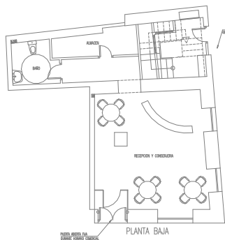
PLANTA BAJA
